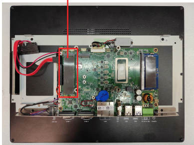
貼附 M.2 Thermal pad
