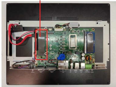
贴附 M.2 Thermal pad
